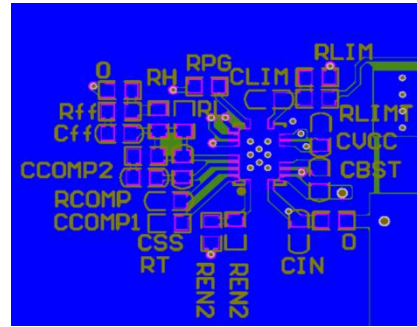
Figure18. Bottom Layer
