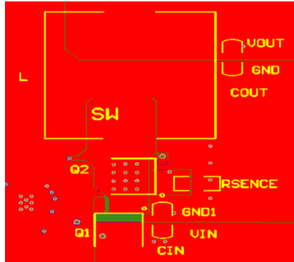
Figure17. Top Layer
